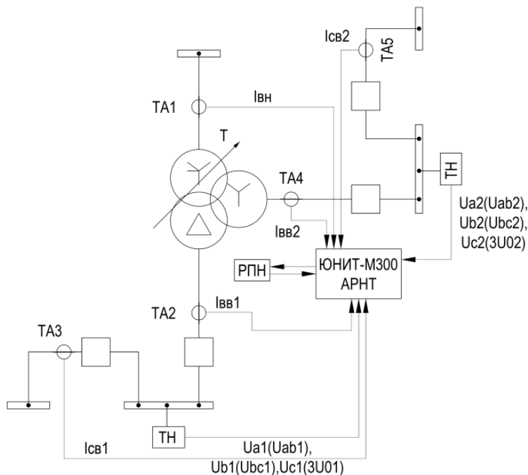
Рисунок 2.2 – Подключение аналоговых цепей устройства для схемы с трехобмоточным трансформатором
